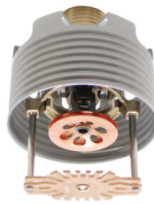
RC-RES 3.7K (SS8261)
