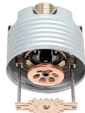
RC-RES 5.8K (SS8561)
