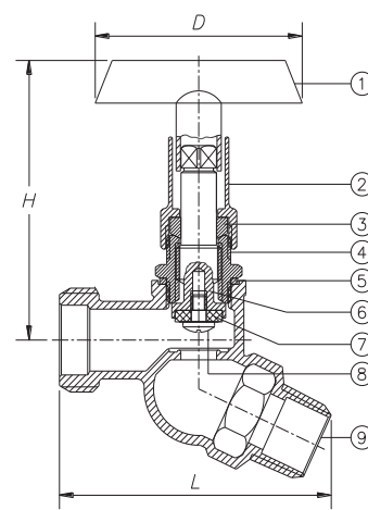
1/2" MIP
